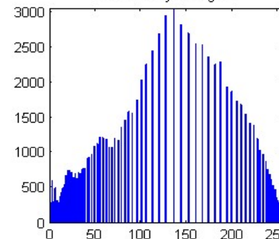
Ekvalizovaný histogram
