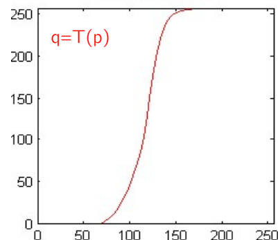
Transformační fce
