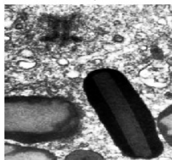
Ekvalizovaný obrazek
