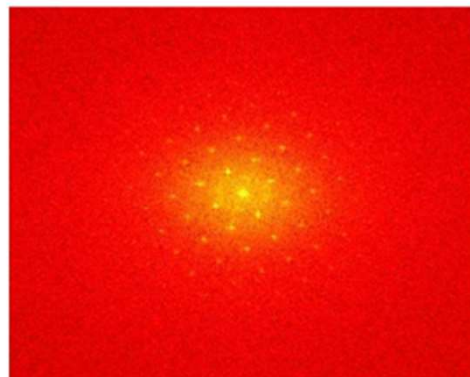
|F(u,v)|
